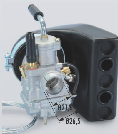
CP POLINI WITH FILTER, CLAMP CONNECTION FOR VESPA 50 (INTAKE MANIFOLD 16/16) POLINI CP CON FILTRO, ATTACCO A FASCETTA PER VESPA 50 COLLETTORE 16/16
